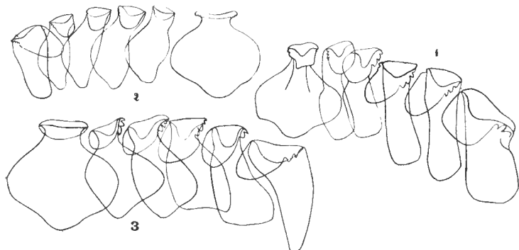
FIG. 1. Gibbula pennanti , Radula \times 450 \times 1/3 ; FIG. 2. Gibbula rarilineata , Radula \times 450 \times 1/3 ; FIG. 3. Gibbula richardi , Radula \times 450 \times 1/3 .
